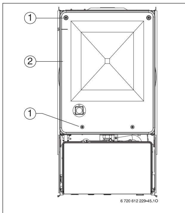
72. attēls. Gaisa kastes atvēršana
