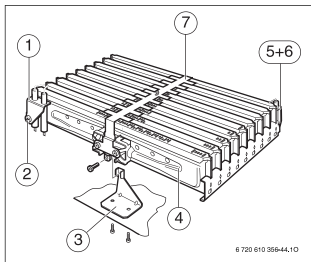
74. attēls. Degļu bloks
