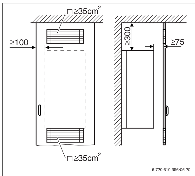
8. attēls. Gaisa pieplūdes atveres, iebūvējot iekārtu skapī
