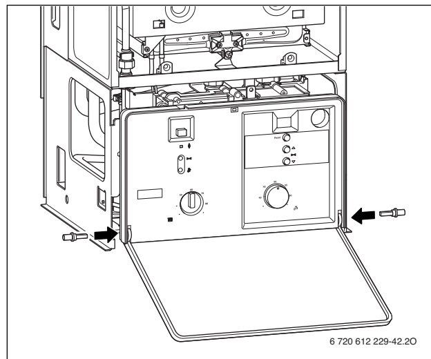
12. attēls. Vāka montāža
