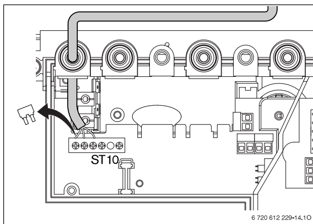
15. attēls. Easyswitch pieslēgšana
