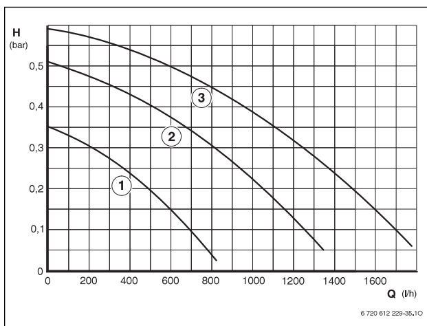
33. attēls. Sūkņa raksturīkne iekārtai Logamax U052-24/28
