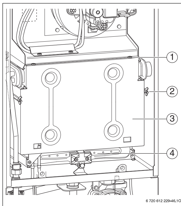
73. attēls. Degkammeras atvēršana
