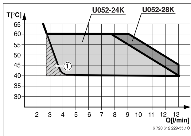
28. attēls. Diagramma ar aukstā ūdens ieplūdes temperatūru +15 °C
