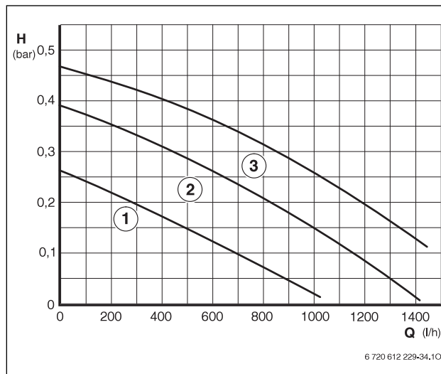
32. attēls. Sūkņa raksturīkne iekārtai Logamax U052-24/28K
