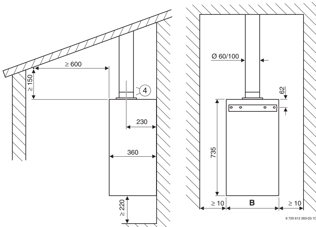
5. attēls. Slīps jumts
