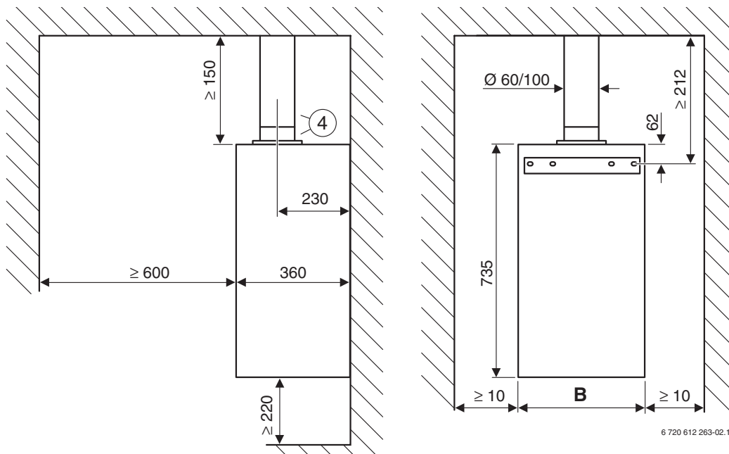
4. attēls. Horizontāls jumts
