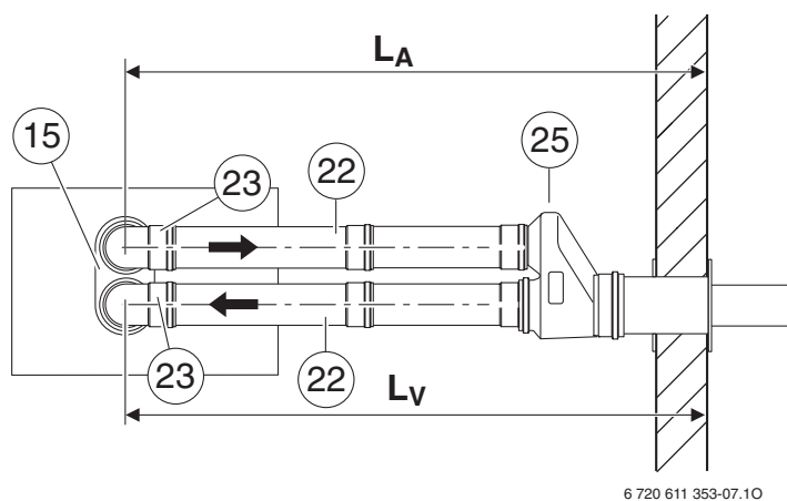
11. attēls. Dūmgāzu novadišana atbilstoši C_{12}
