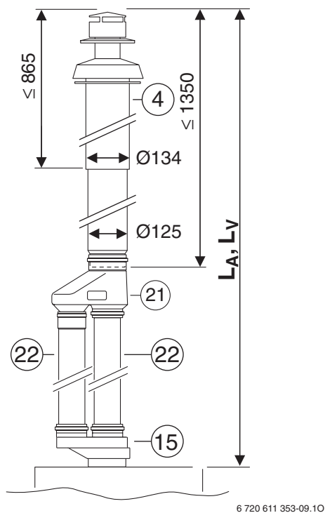
13. attēls. Dūmgāzu novadišana atbilstoši C_{32}
