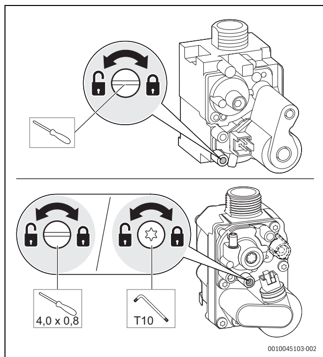
Att. 46 Gāzes pieslēguma spiediena mērīšana
