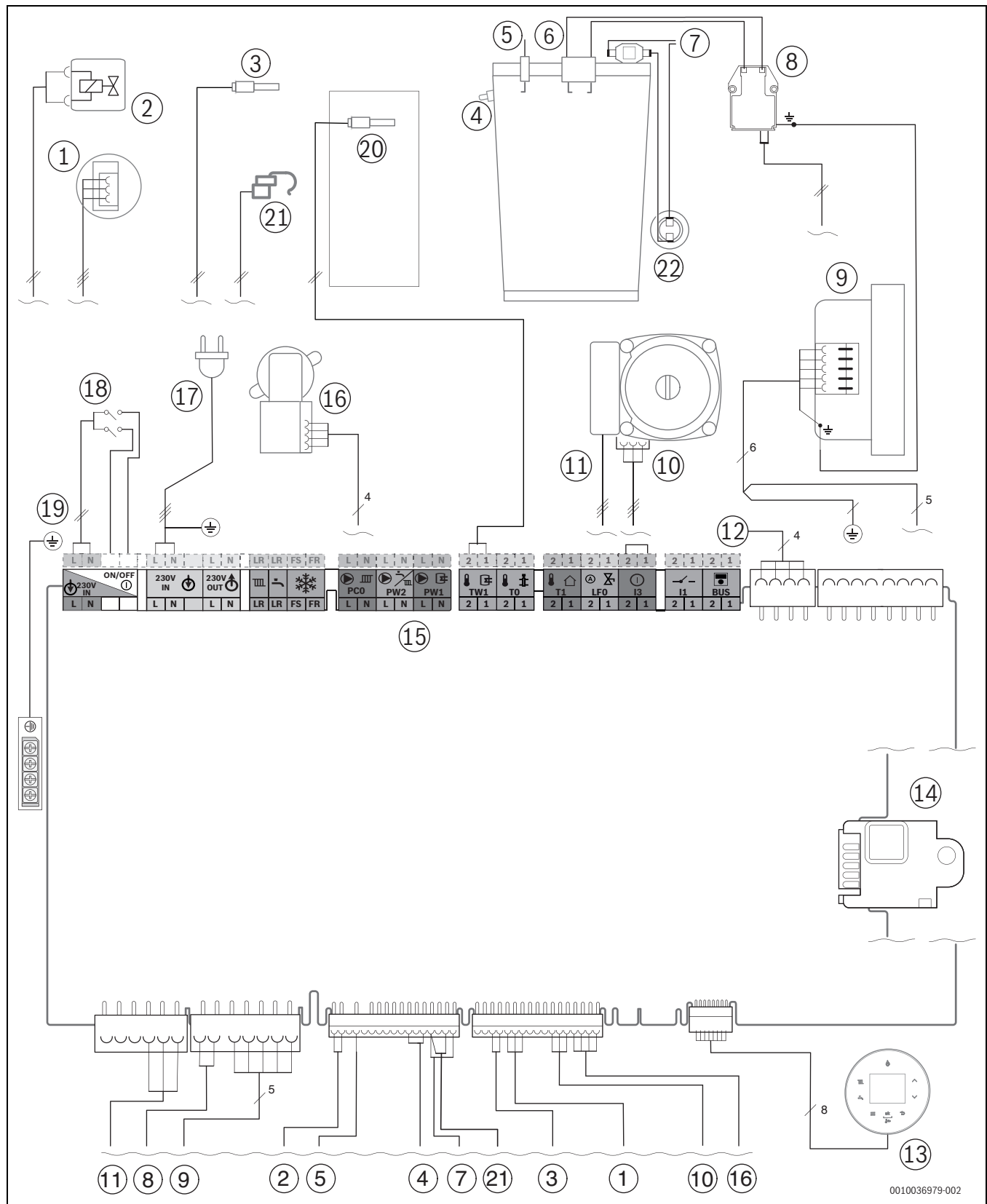
Att. 85 Elektroinstalācija
